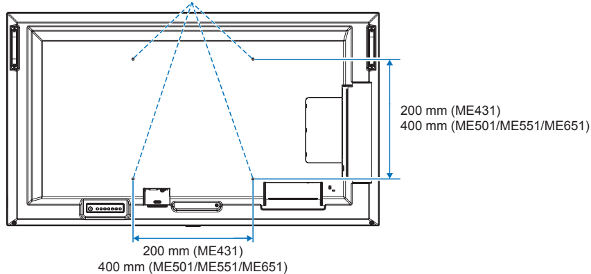
VESA 安装接口 M6 (ME431/ME501/ME551), M8 (ME651)
